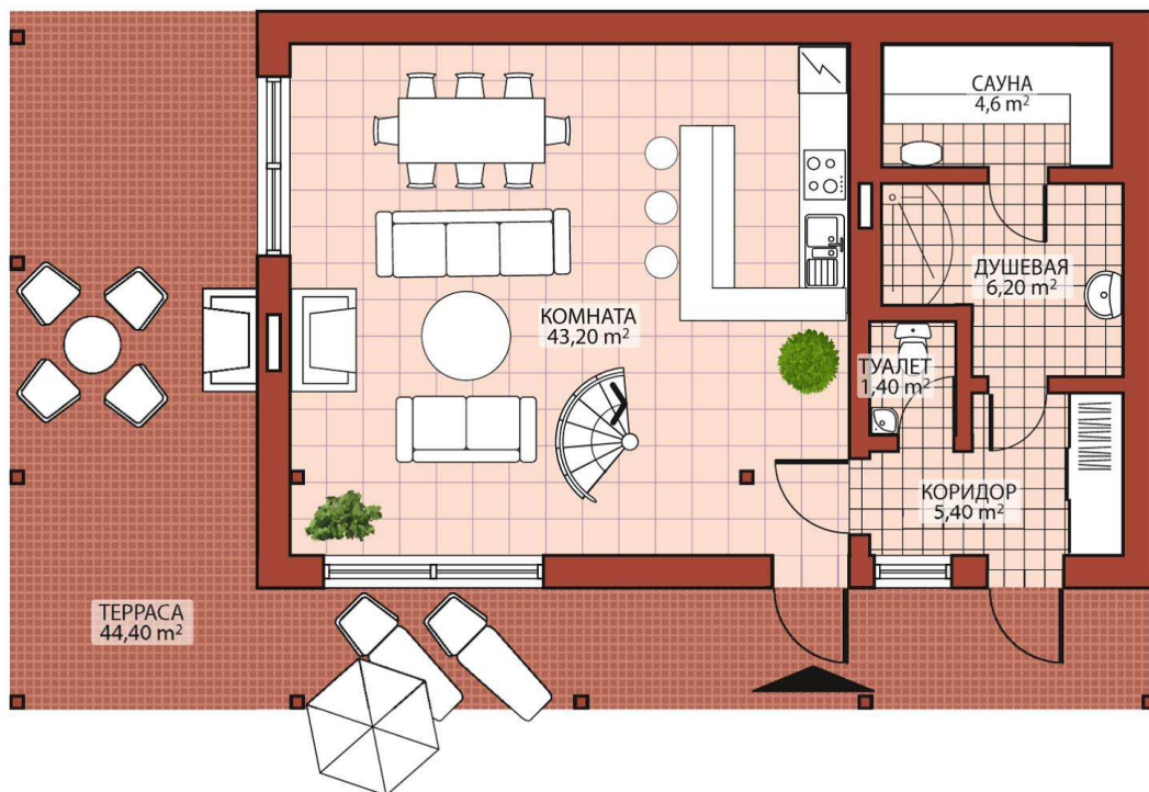
ПЛАН 1-ого ЭТАЖА ГОСТЕВОГО ДОМА
