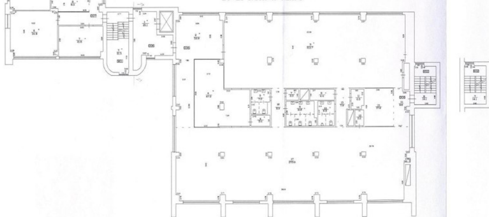
BŪVES 3. STAVA PLĀNS
